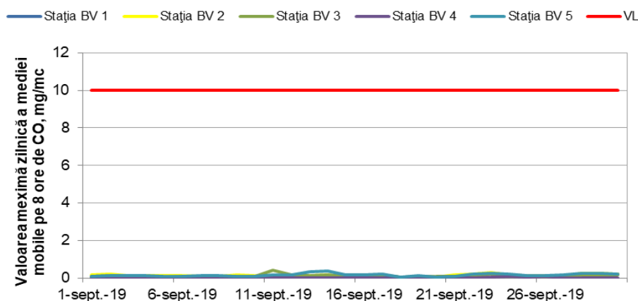
*din motive tehnice (analizor defect) captura de date valide la stația BV4 a fost de 10,1% Figura 1.1.2.5.1. Evoluția maximelor zilnice ale mediei mobile de CO în luna septembrie
