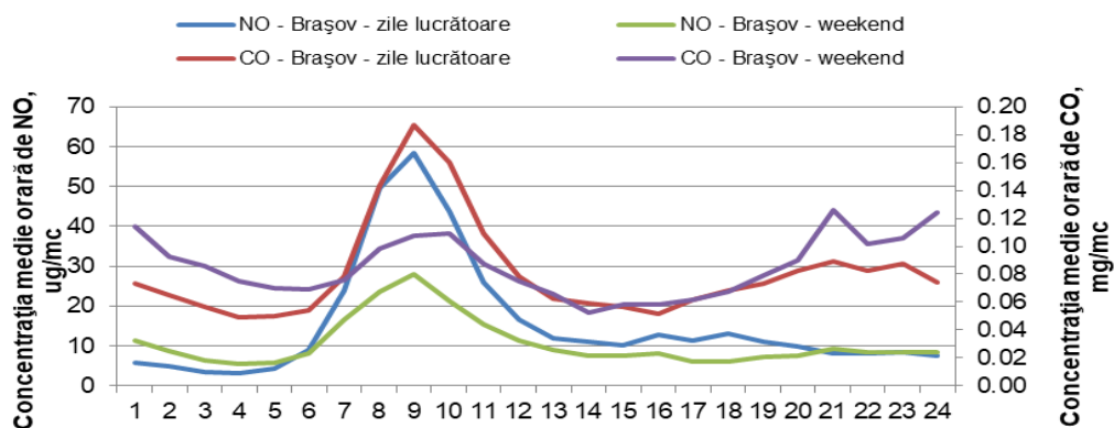
Figura 1.1.2.2.5. Ciclul zilnic al \text{NO} și \text{CO} în timpul săptămânii
