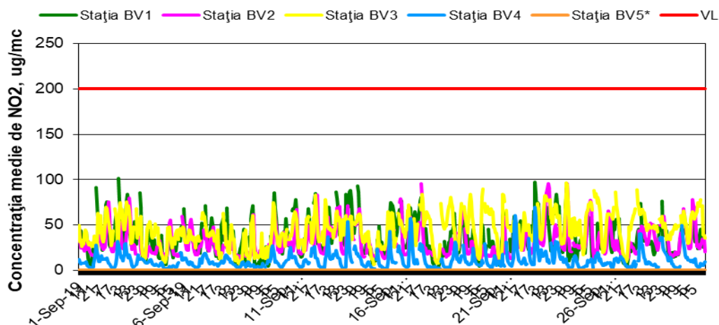
Figura 1.1.2.2.1. Evoluția mediilor orare de NO 2 în luna septembrie
