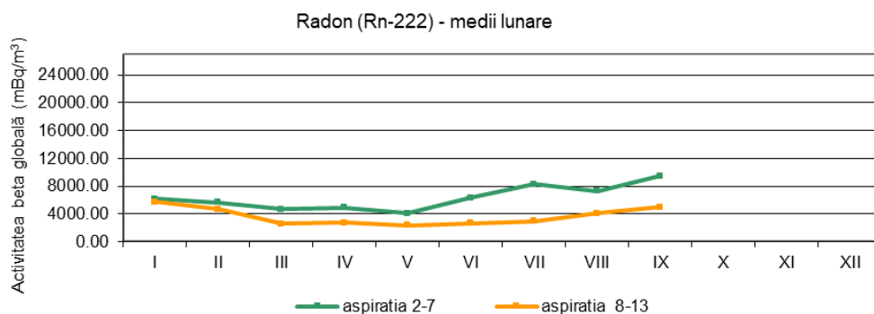
Fig. 1.3.2. Activitatea calculată a Radonului
