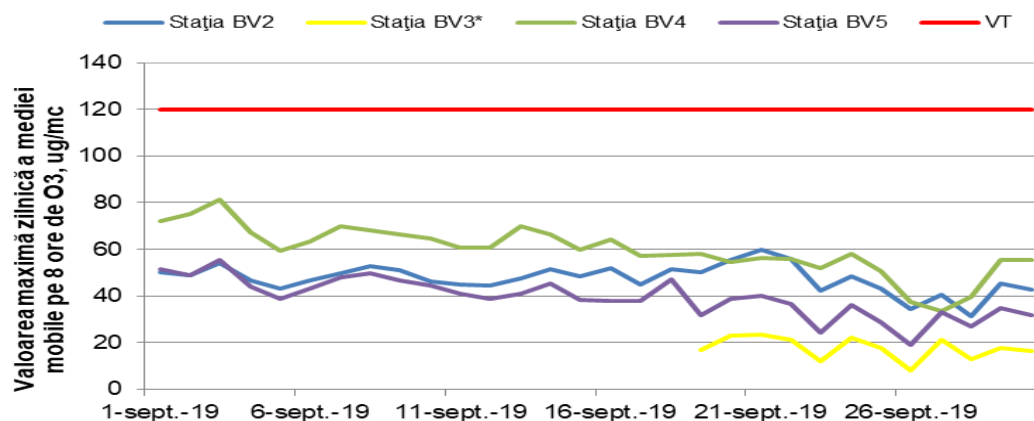
Figura 1.1.2.3.1. Evoluția maximelor zilnice ale mediilor mobile pe 8 ore de O 3 în luna septembrie
