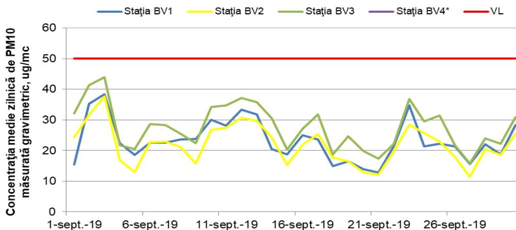
Figura 1.1.2.4.1. Evoluția mediilor zilnice de PM 10 în luna septembrie
