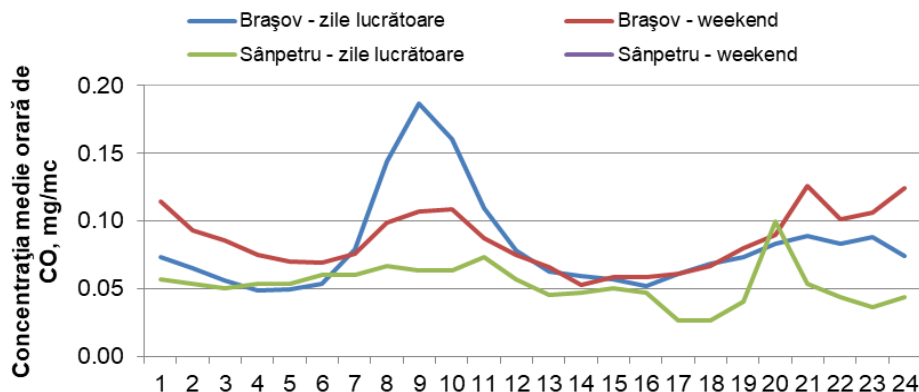
Figura 1.1.2.5.3. Ciclul zilnic al CO în timpul săptămânii
