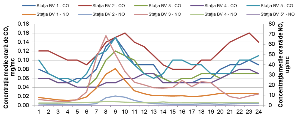
Figura 1.1.2.2.4. Ciclul zilnic al \text{NO} și \text{CO}
