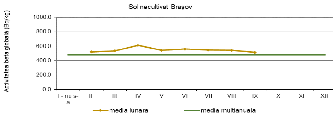
Fig. 1.3.8. Activitatea beta globală la 5 zile pentru solul necultivat
